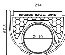
ENDSCHEIBE MIT ABLAUF 200/160
